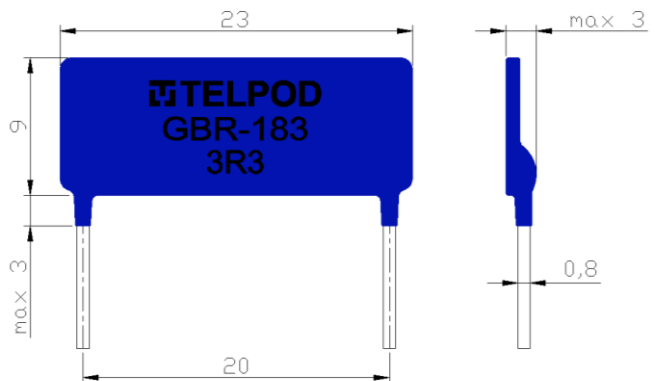
Rys. 1. Wygląd zewnętrzny i wymiary [mm]
